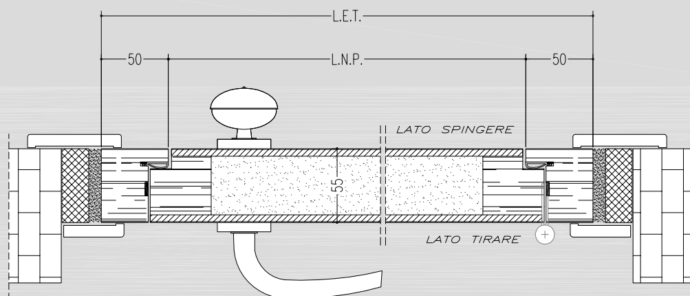
SEZIONE ORIZZONTALE
