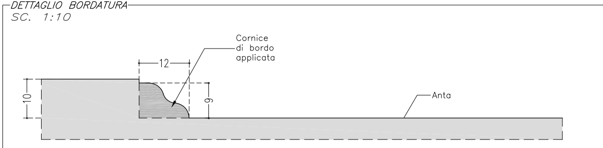
DETTAGLIO BORDATURA + PANNELLO SC. 1:10
