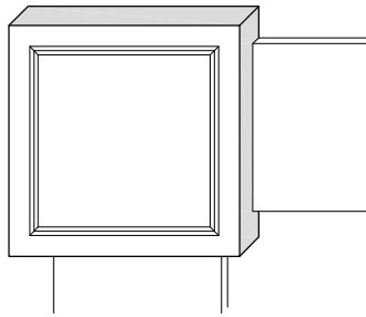
ANG E Sezione: 110x110x26 mm
