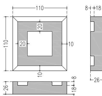
ANG E Sezione: 110x110x26 mm
