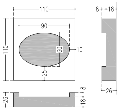
ANG D Sezione: 110x110x26 mm
