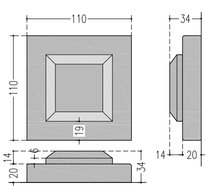
ANG F Sezione: 110x110x34 mm
