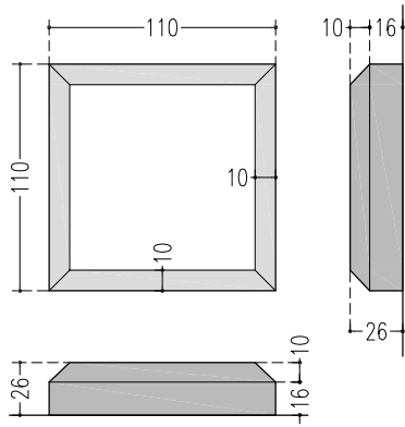
ANG SA Sezione: 110x110x26 mm
