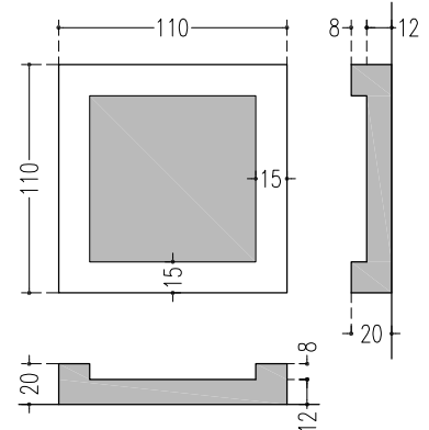
ANG RC Sezione: 110x110x20 mm
