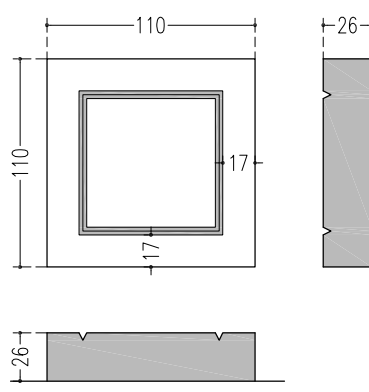
ANG BB Sezione: 110x110x26 mm
