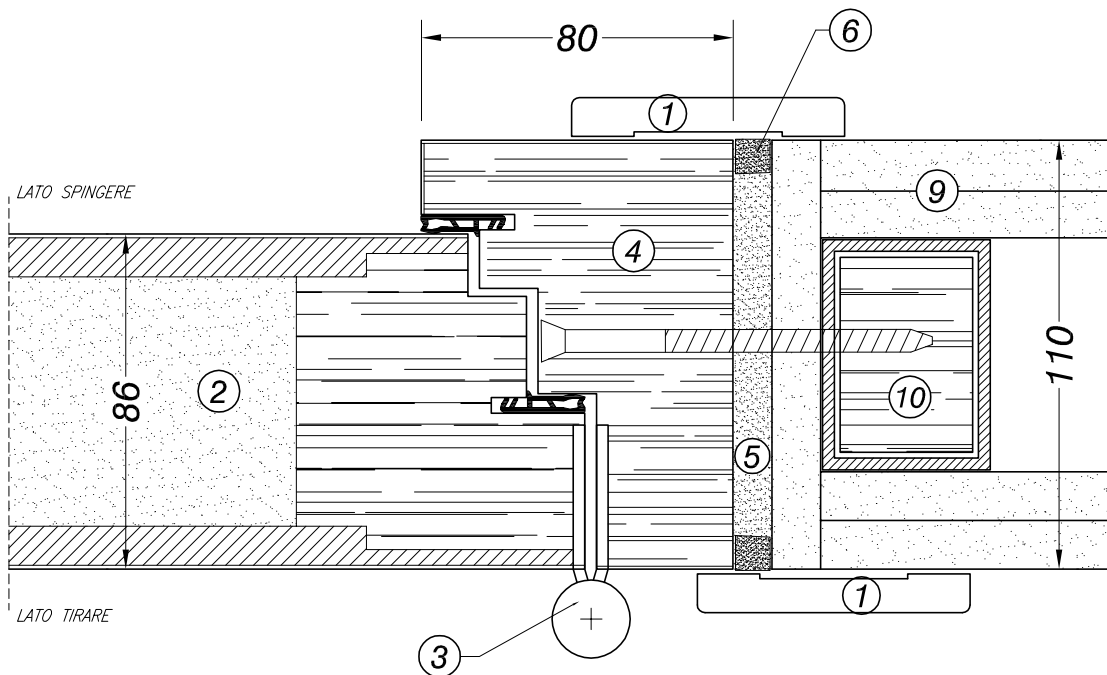
DETTAGLIO TELAIO-ANTA - MONTAGGIO SU CARTONGESSO
