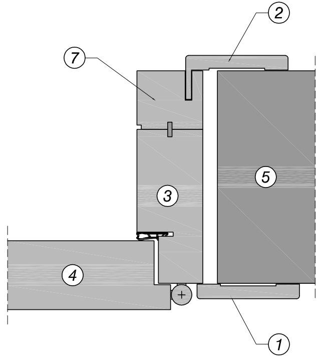
POSIZIONAMENTO GENERICO PORTA CON BATTUTA VERSIONE OPZIONALE CON IMBOTTE RINGROSSATA
