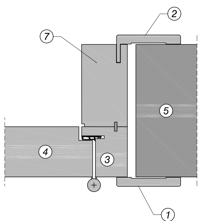
POSIZIONAMENTO GENERICO PORTA COMPLANARE VERSIONE OPZIONALE CON IMBOTTE RINGROSSATA
