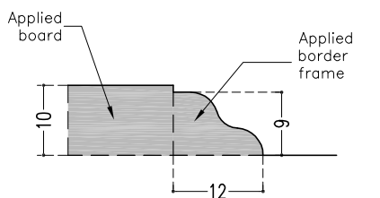
BORDER DETAIL—SC. 1:10
