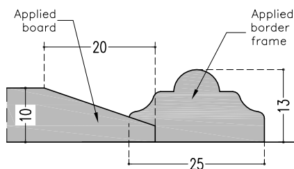
BORDER DETAIL—SC. 1:10
