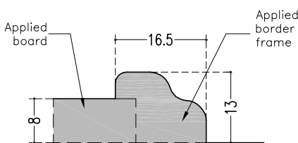
BORDER DETAIL—SC. 1:10
