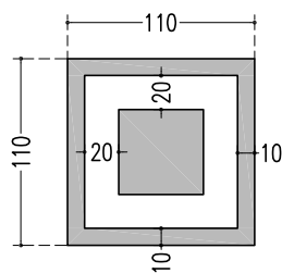
ANG E Section : 110 x 110 x 26 mm
