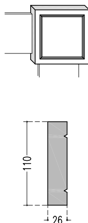
ANG BB Section : 110 x 110 x 26 mm
