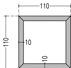
ANG SA Section : 110 x 110 x 26 mm
