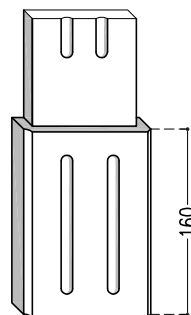
PD FD Section : 110 x 25 x 160 mm
