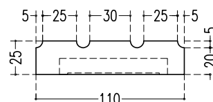
PD FD Section : 110 x 25 x 160 mm
